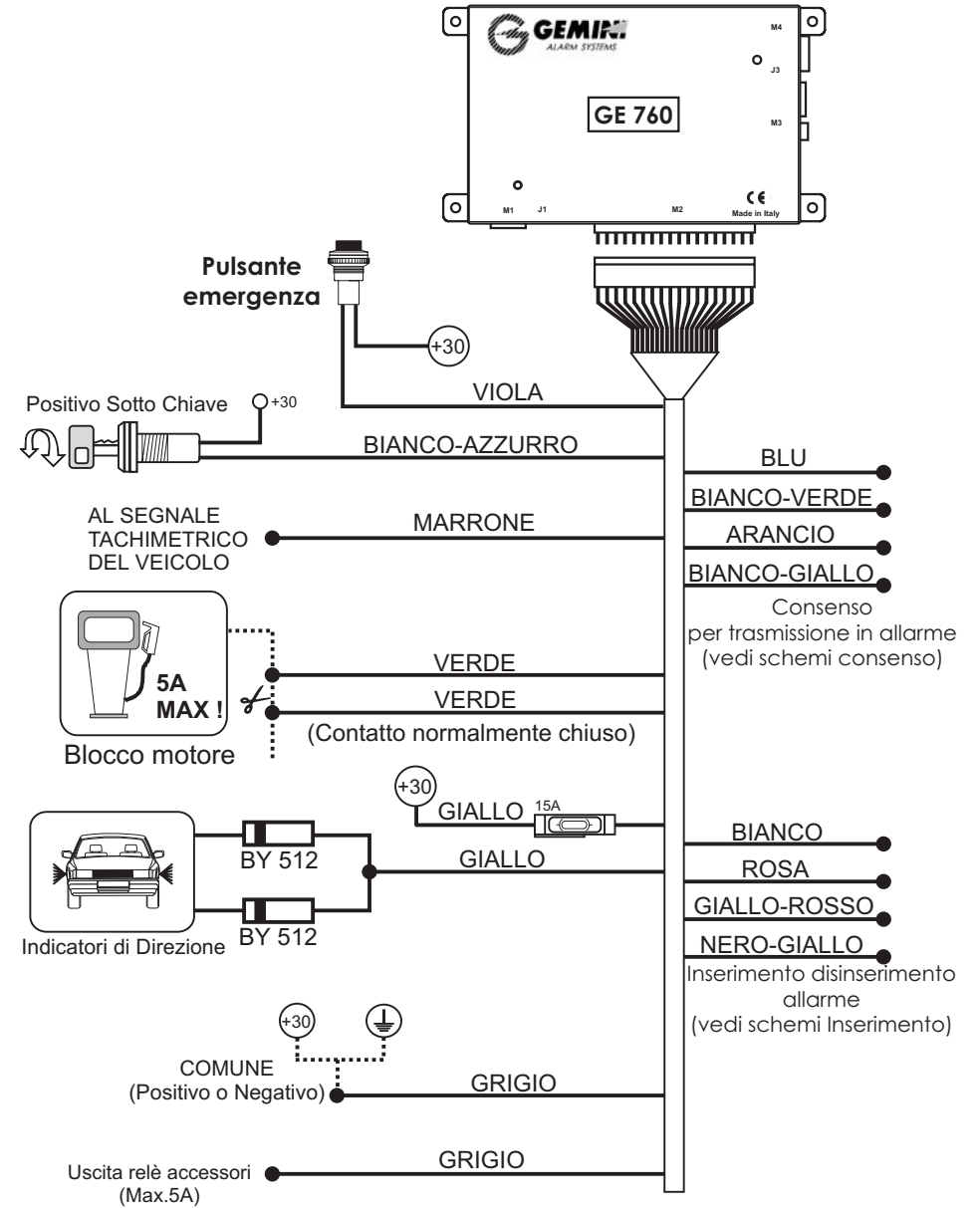
Schema di collegamento con il veicolo
